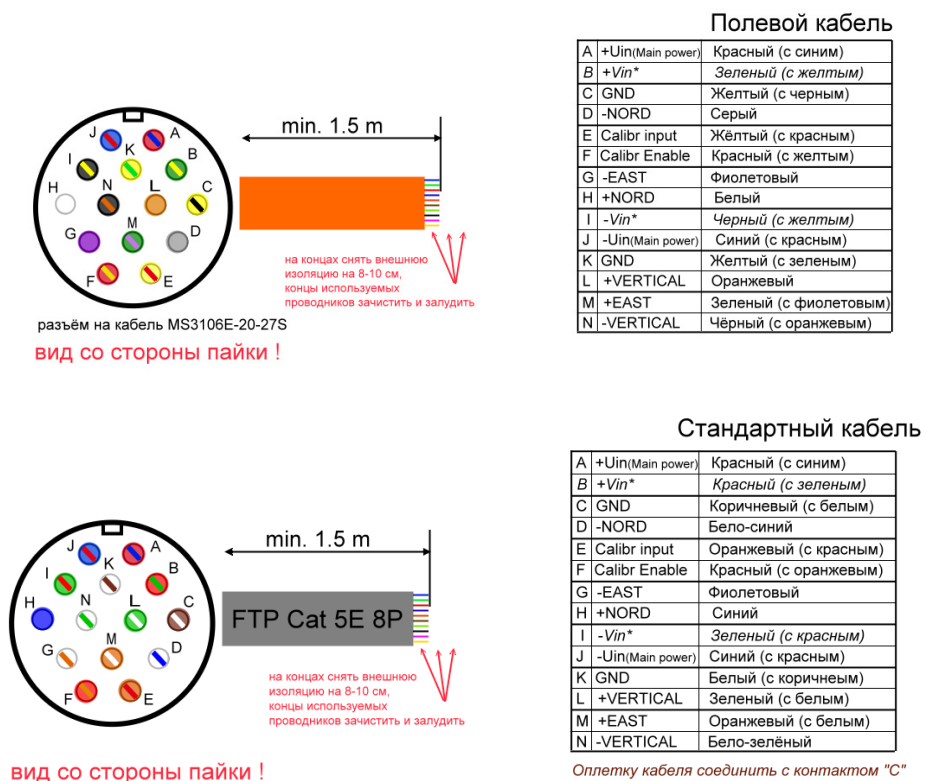
Рис. 2б. Схема распайки разъема сейсмометра СМЕ-6211
