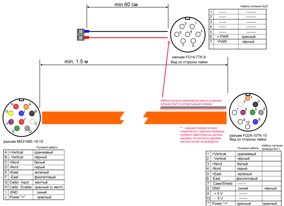
Рис. 2а. Схема полевого кабеля сейсмометра СМЕ-6211 в составе сейсмостанции Байкал-СМЕ
