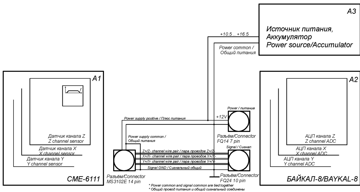
Рис. 16. Типовая схема соединений сейсмометра CME-6111 в составе сейсмостанции Байкал-CME (продолжение)
